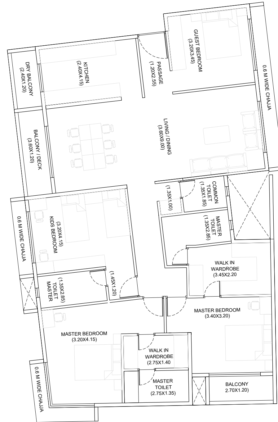
4BHK UNIT B 160 SQ. M.
